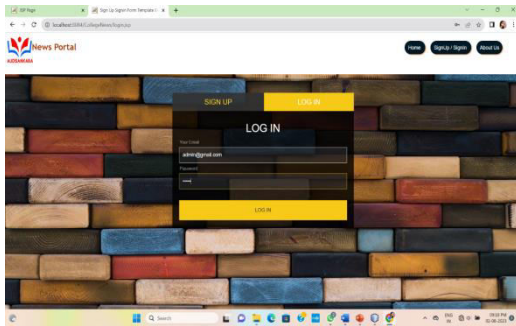
Fig. 3: Login Page
