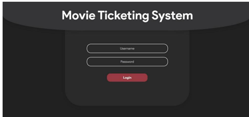
FIG1 : HOME SCREEN
